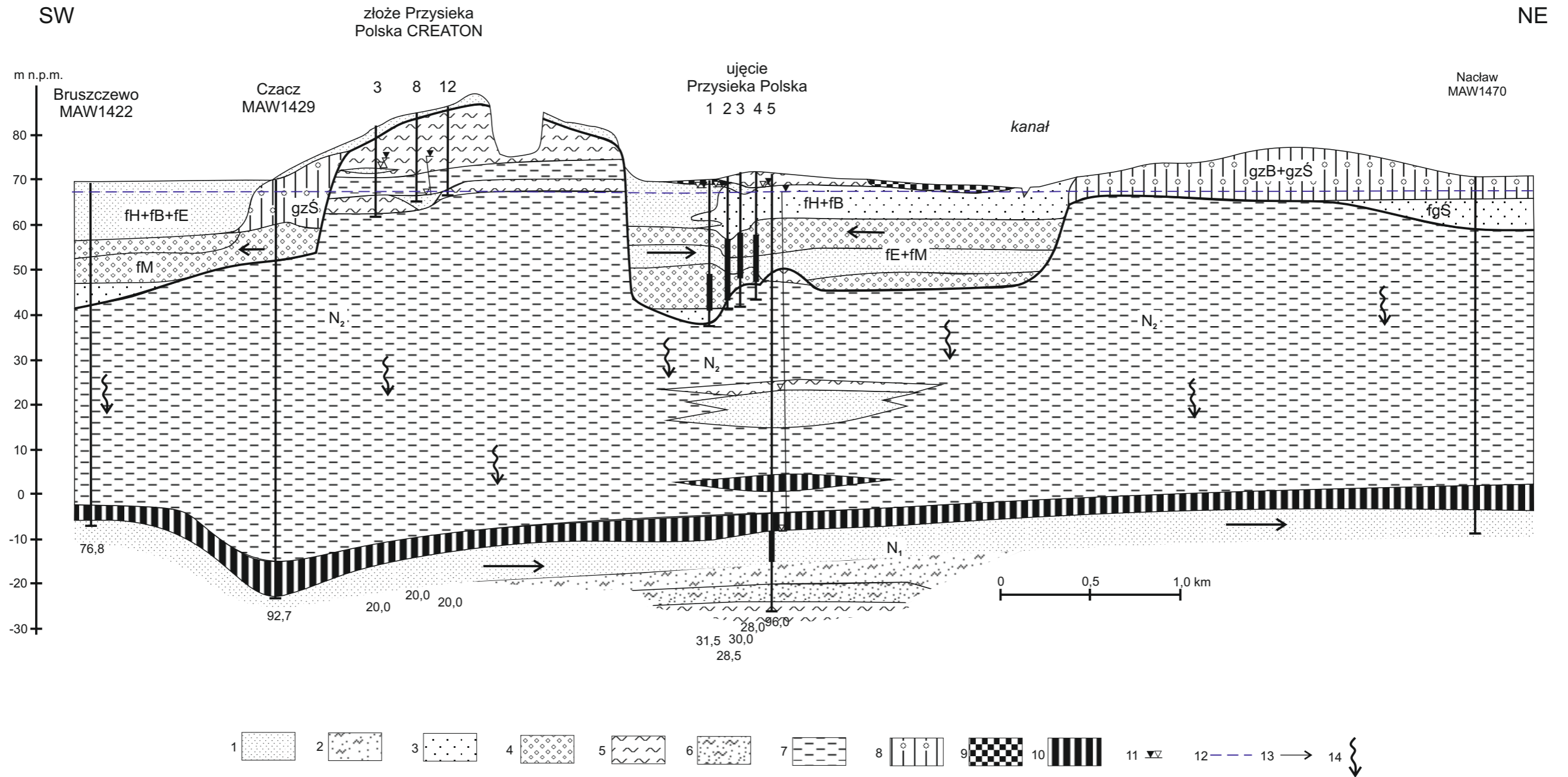
Załącznik 4. Przekrój hydrogeologiczny A - A
